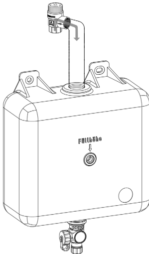
Figura 2: Montare cu conductă de evacuare și container de colectare specific pentru instalații solare
