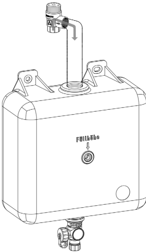
Figure 2: Montage avec conduite de décharge et collecteur liquide solaire
