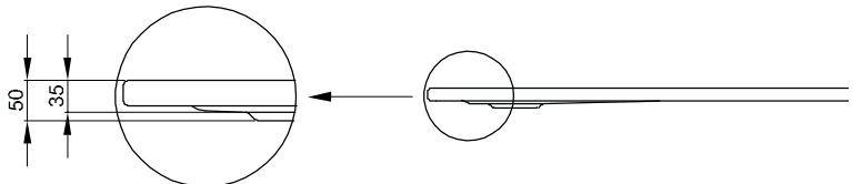
Duschwannen mit Schenkel > 1000 mm
